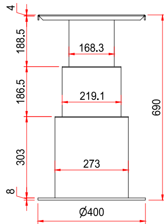
PROSPETTO APERTO scala 1:10
